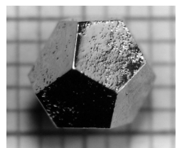
Un quasi-cristal dodécacédral, formé de Holmium, Magnésium et Zinc
